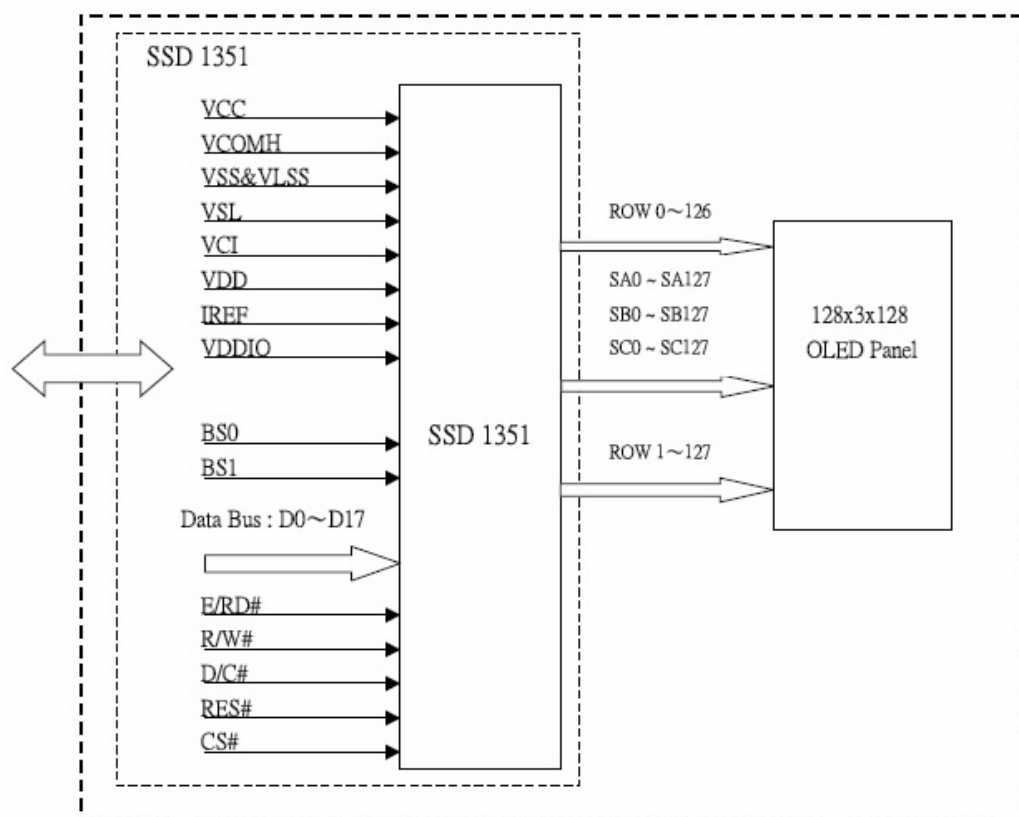
RiTdisplay 128x3x128 OLED Module
