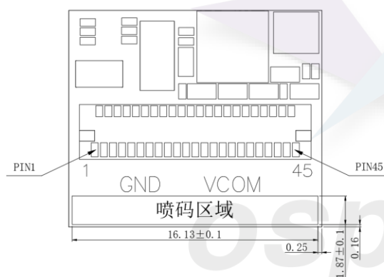
背视图
