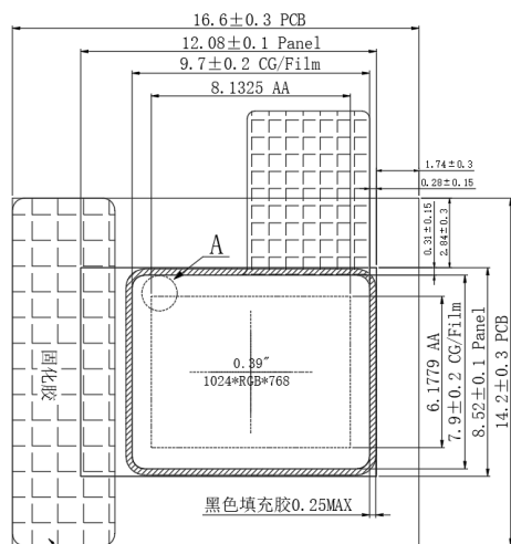
主视图
